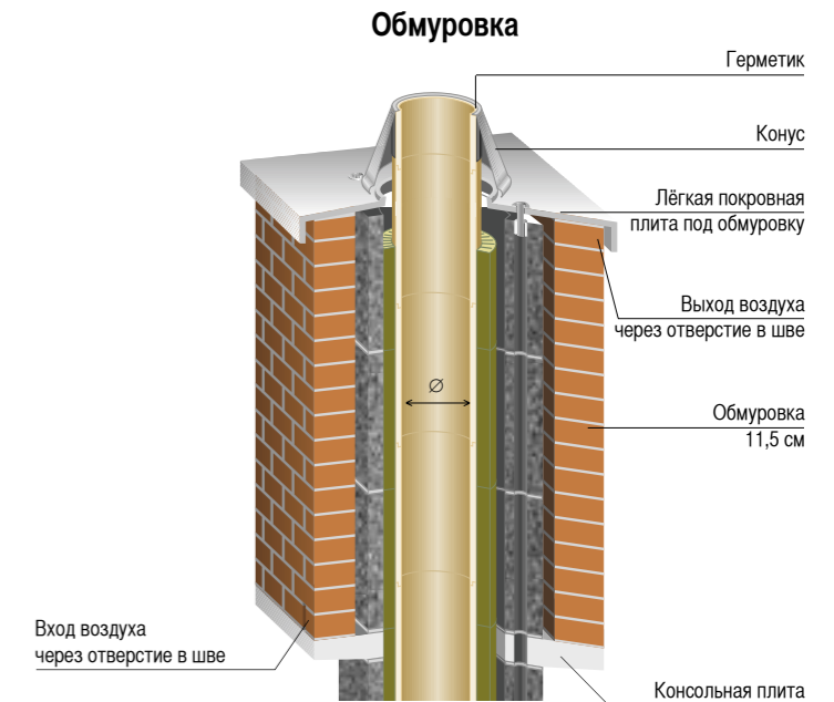
Выполняемая по месту обмуровка на консольной плите
