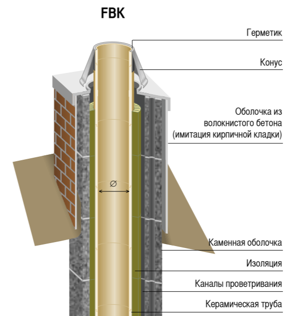
Оболочка дымовой трубы из волокнистого бетона с имитацией кирпичной кладки
