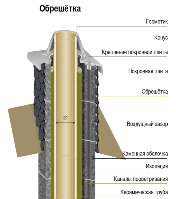
Выполняемая по месту обрешётка
